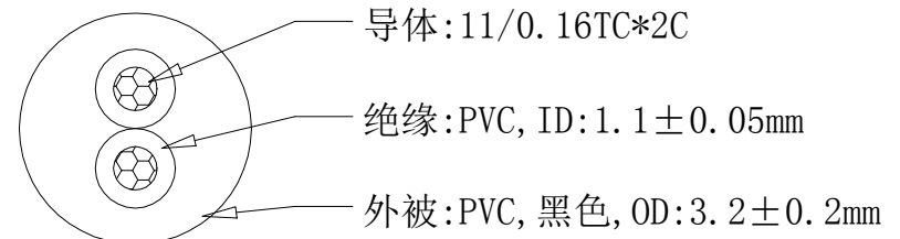
截面图
