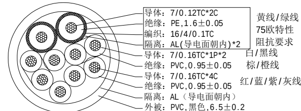
截面图
